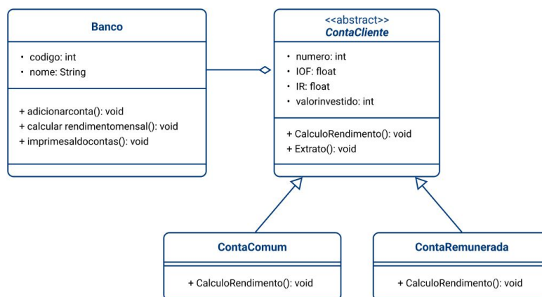
Diagrama de classes abstratas.
